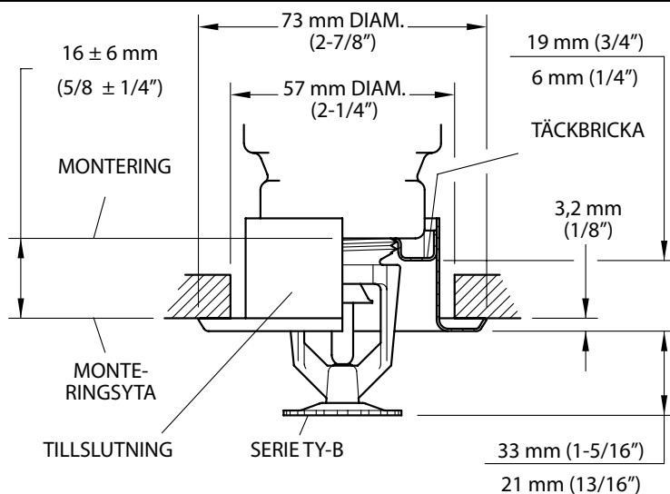
BILD 5 SERIE TY-B INSÄNKTA PENDENTSPRINKLERS 19 mm (3/4") TOTAL JUSTERING TYP 10 I TVÅ DELAR MED INSÄNK TÄCKBRICKA K80, 1/2" NPT
